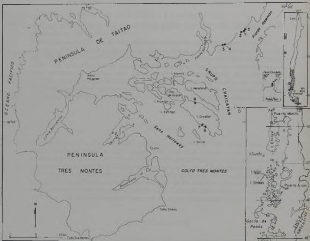
Figura 1. Ubicación de las localidades fosilíferas con Glycymeris ( Glycymeris ) taitaoensis sp. nov. en la costa occidental de Fierdo Newman y en Isla Crosslet, en el interior de Golfo Tres Montes (Aisen, Chile Austral). 1: 140984.4 (material tipo); 2: 091083.3; 3: 140984.1; 4: 140984.2; 5: 140984.5; 6: 060984.3; 7: 070984.1; 8: 090984.2.
