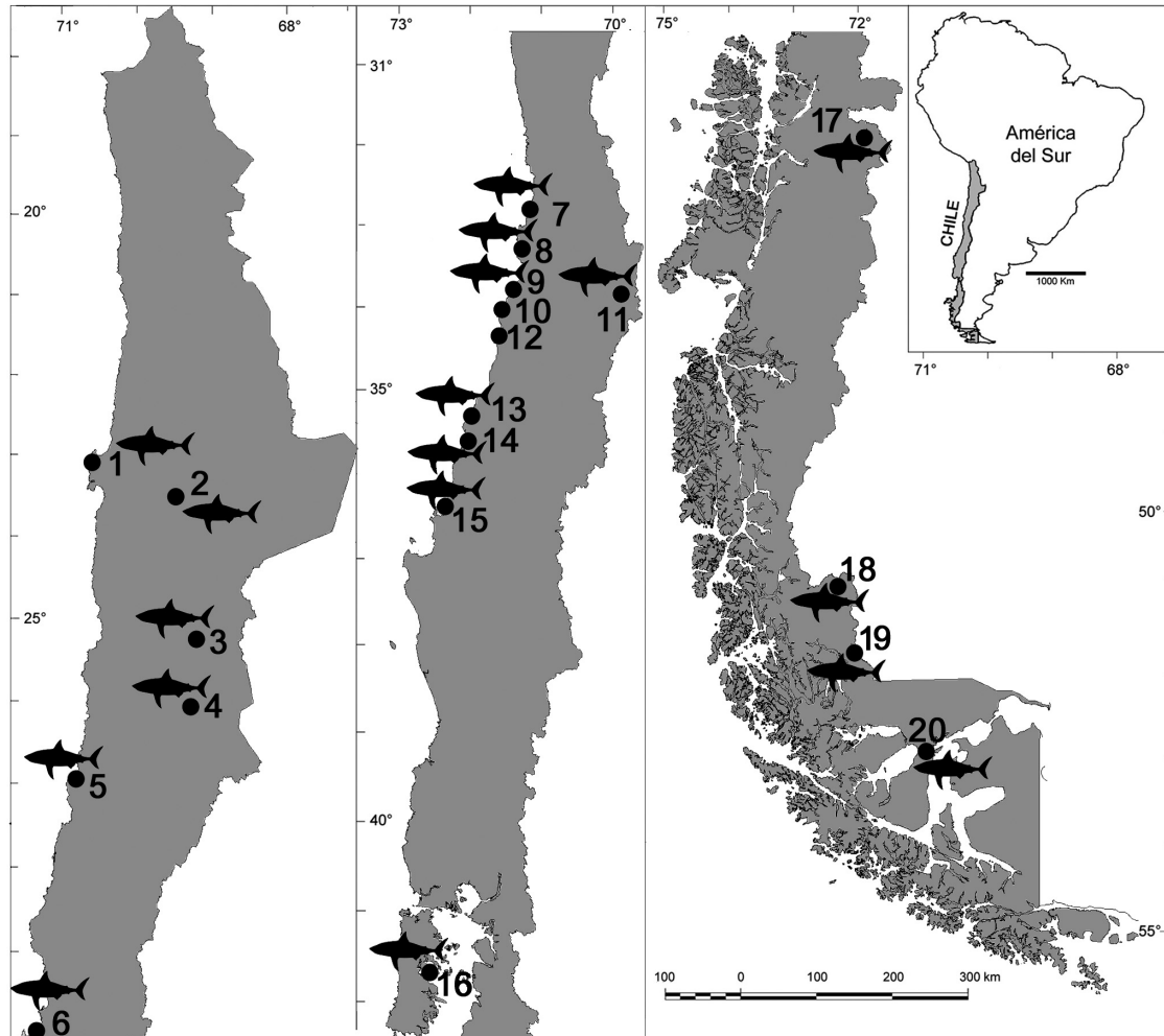
FIGURA 1. Mapa mostrando principales localidades y unidades fosilíferas con peces condrictios en Chile. 1) La Portada y Caleta Herradura de Mejillones, Región de Antofagasta. Formación la Portada, Mioceno Medio-Plioceno. 2) Cerro Negro, Región de Antofagasta. Formación Peine?, Pérmico. 3) Punta del Viento, Región de Antofagasta. Formación Punta del viento, Triásico (Rético). 4) La Coipa, Región de Atacama. Estratos de Mono, Triásico. 5) Caldera, Región de Atacama. Formación Bahía Inglesa. Mioceno Superior y Plioceno inferior. 6) Coquimbo, Región de Coquimbo. Formación Coquimbo, Mioceno-Plioceno. 7) Horcón, Región de Valparaíso. Formación Horcón, Plioceno. 8) Algarrobo, Región de Valparaíso. Estratos de la Quebrada Municipalidad, Maastrichtiano; Estratos de Algarrobo, Eoceno medio-superior. 9) Lo Abarca, Región de Valparaíso. Formación Lo Abarca, Mioceno Superior. 10) Navidad-Matanzas, Región de O'Higgins. Formación Navidad, Mioceno Inferior. 11) Lo Valdés, Región Metropolitana. Formación Lo Valdés, Jurásico Superior (Titaniano superior). 12) Punta Topocalma. Formación Punta Topocalma, Campaniano-Maastrichtiano. 13) Caleta Loanco, Región del Maule. Formación Quiriquina, Maastrichtiano superior. 14) Distintas localidades en la costa de la Región del Biobío, Formación Quiriquina, Maastrichtiano superior. 15) Cerro San Miguel, Talcahuano, posiblemente Formación Cosmito o equivalente, Paleoceno. 16) Isla de Chiloé, Región de los Lagos? Estratos de Chonchi, Oligoceno-Mioceno. 17) Región de Aysén, Formación Apeleg, Cretácico Inferior. 18) Sierra Baguales, Región de Magallanes. Formación Dorotea, Maastrichtiano; Formación Río Baguales (=Man Aike), Paleoceno?- Eoceno superior. 19) Cerro Dorotea, Puerto Natales, Región de Magallanes. Formación Dorotea, Maastrichtiano superior. 20) Río de Las Minas, Península de Brunswick, Región de Magallanes. Formación Loreto, Eoceno superior (Priaboniano).
