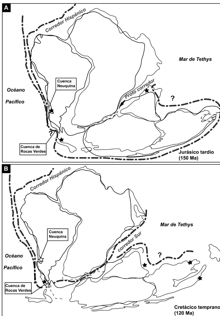
FIGURA 17. Esquema paleogeográfico del límite Jurásico - Cretácico: A) Jurásico superior (150 Ma. aprox.). Hacia fines del Titiánico o Berriasiano temprano el Corredor Hispánico habría conectado a las faunas del hemisferio norte con el sur. El corredor de Sudáfrica y Rocas Verdes ('South African / Rocas Verdes Corridor') en el hemisferio sur ya habría comenzado a formarse, pero no habría sido completamente efectivo aún. El aislamiento producido en el hemisferio sur habría permitido la especialización del grupo. B) Cretácico temprano (120 Ma. aprox.). Ictiosaurios del hemisferio sur se conectarían con fauna del Tethys oriental a través del ya efectivo corredor de Sudáfrica y Rocas Verdes ('South African /Rocas Verdes Corridor'), mientras que el Corredor Hispánico pudo haber continuado actuando como paso para fauna marina en el hemisferio norte. Estrellas indican localidades donde han sido encontrados ictiosaurios ophthalmosauridos. La estrella blanca indica P. hauthali en la Cuenca Neuquina y de Rocas Verdes. Líneas punteadas oscuras indican las posibles rutas de dispersión de ophthalmosauridos. Imagen modificada de Riccardi (1991).
