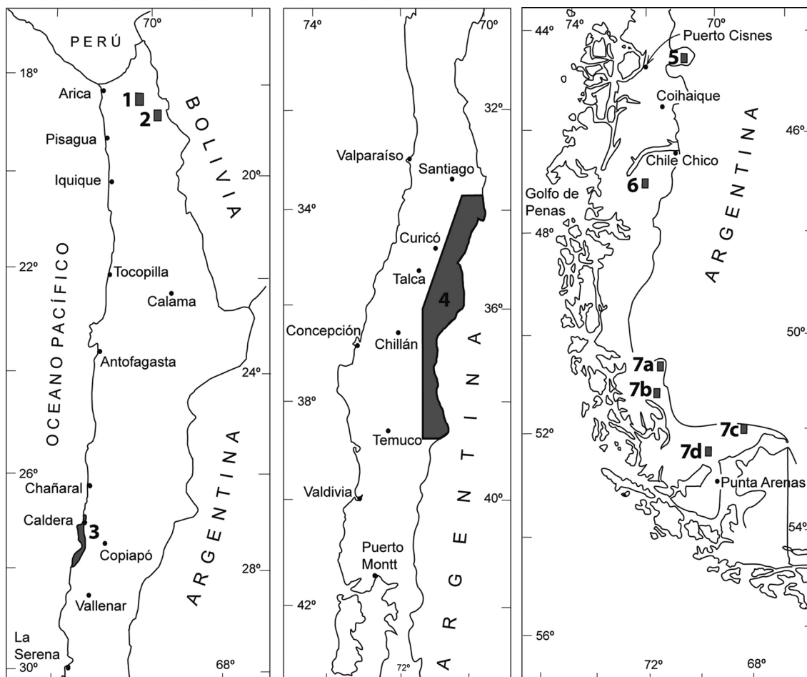
FIGURA 1. Mapa de ubicación de las localidades y regiones donde se han encontrado restos de mamíferos en rocas cenozoicas pre-pleistocénicas (terciarias) en Chile: 1. Caragua en la Precordillera oriental de Arica, 2. Chucal, en la parte oriental de la Cordillera Occidental de Arica, 3. Franja costera de la región de Caldera, Región de Atacama, 4. Cordillera Principal de Chile central, 5. Río Cisnes (ex Frías), en la región fronteriza de Aysén, 6. Pampa Castillo en la Meseta Guadal-Cosmelli, al sur del Lago General Carrera, Aysén, 7. Región de Magallanes: a. Alto río Baguales, b. Lago Toro, c. Cueva de Fell, y d. Sector de Laguna Blanca.
