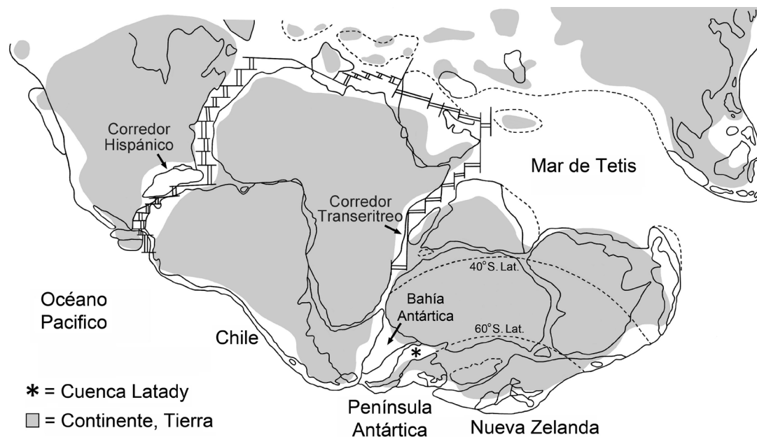
FIGURA 12. Mapa paleogeográfico de la Tierra durante el Jurásico Medio-Superior mostrando la posición probable de Chile, el Grupo Latady en la Península Antártica y el Corredor Hispánico uniendo al Paleopacífico y el Mar de Tetis (ligeramente modificado de Arratia y Hikuroa 2010).
