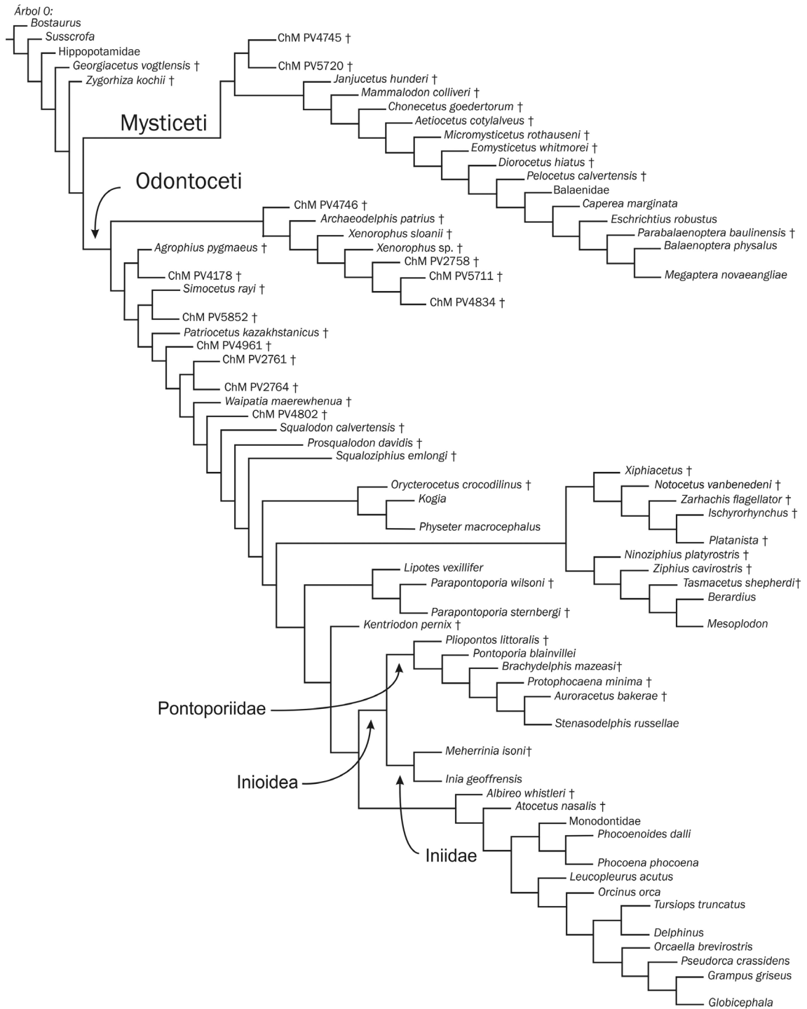
FIGURA 2. Hipótesis de relación filogenética en Cetacea, con énfasis en odontocetos. Modificado de Geisler et al. 2012.
