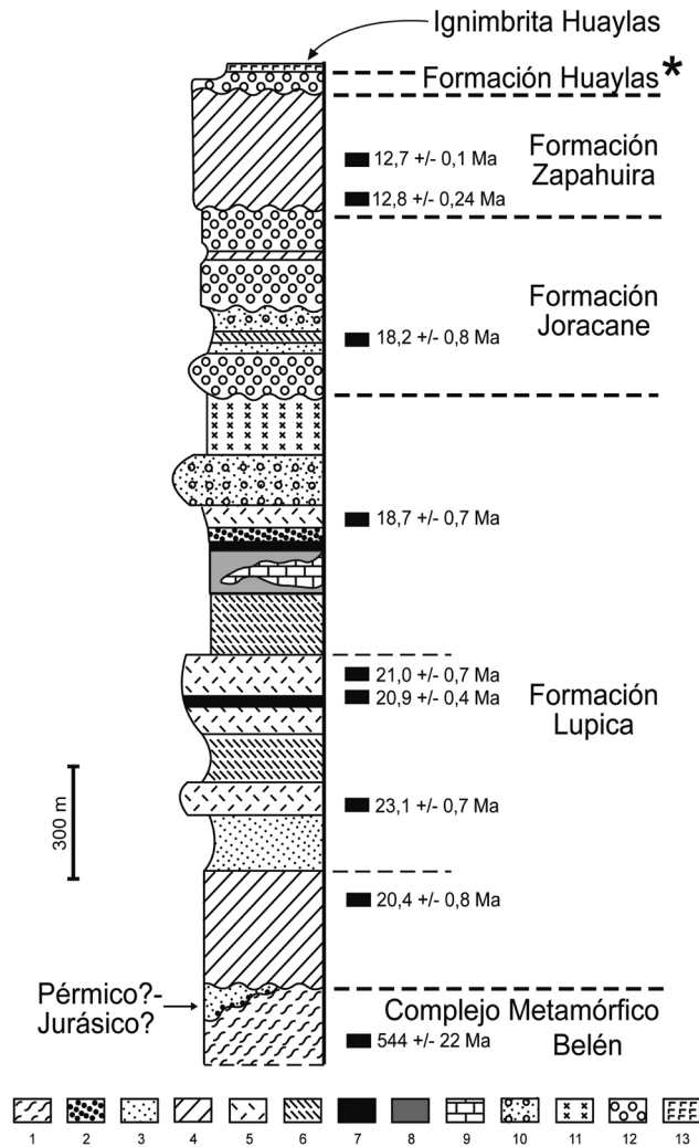
FIGURA. 3. Columna estratigráfica de la Precordillera oriental de Arica con indicación de las edades radioisotópicas obtenidas en los diferentes niveles (basada en García, 2002, Fariás et al. 2005, Basei et al. 1996). En esta región la unidad fosilífera es la Formación Huaylas (con asterisco). La Formación Lupica se considera un equivalente oriental de la Formación Chucal y se extiende hacia la Cordillera Occidental donde subyace a los depósitos fosilíferos de la Formación Oxaya y se extiende hacia la Cordillera Occidental donde subyace a los depósitos fosilíferos de la Formación Chucal (ver Figura 5). 1. Complejo Metamórfico Belén, 2. Conglomerado basal, 3. Arenisca, 4. Andesita basáltica, 5. Ignimbrita, 6. Toba andesítica, 7. Limolita laminada, 8. Fangolita, 9. Caliza, 10. Arenisca conglomerádica, 11. Toba silícea, 12. Conglomerado, 13. Ignimbrita Huaylas.
